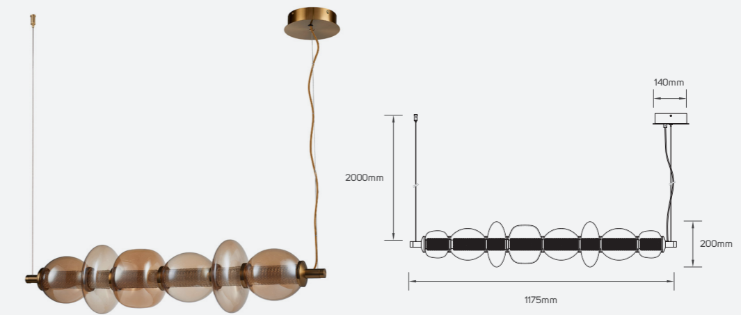
● 661705 24W
