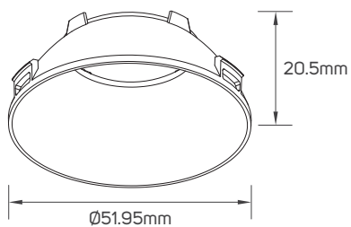
● 613521 - ● 613522 - ● 613523 - ● 613524 - Reflector
