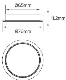
613533 - Frame
