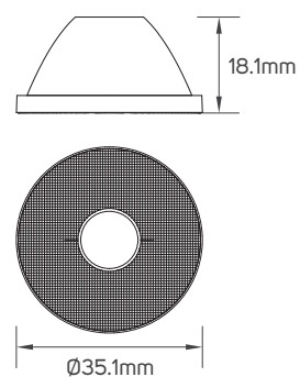
613541 - 613542 - Lens
