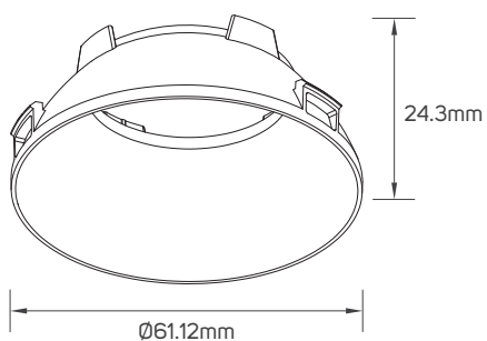
● 613525 - ● 613526 - ● 613527 - ● 613528 - Reflector
