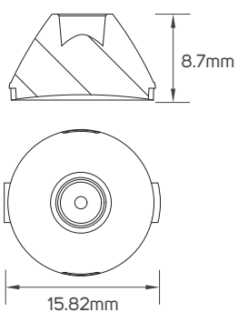
613536 - 613537 - Lens
