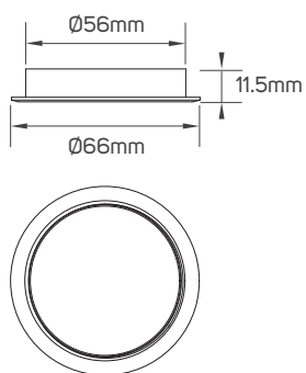
613532 - Frame
