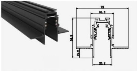
Size:72X54.9X26.3mm
